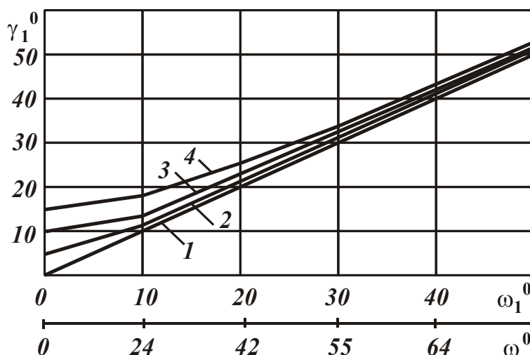
Рис. 5. Зависимость угла \gamma_1 от угла \omega_1 (угла \omega ): 1 - \gamma = 0^0 ; 2 - \gamma = 5^0 ; 3 - \gamma = 10^0 ; 4 - \gamma = 15^0
