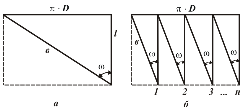
Рис. 2 – Схема рабочей поверхности развертки с одним (а) и с n (б) зубьями, расположенными под углом наклона \omega
