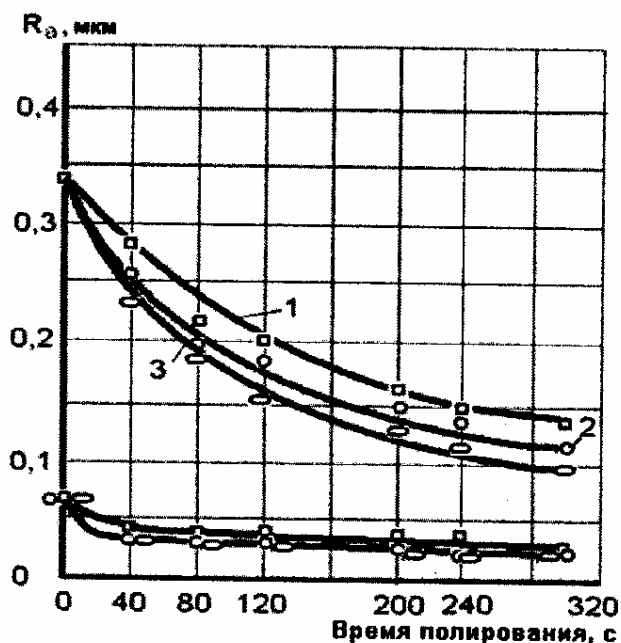
Рис. 1. Зависимость шероховатости поверхностей образцов из стали марки 12×18Н10Т от времени полирования при исходной шероховатости 0,34 и 0,065 мкм: 1 – М3; 2 – М14; 3 – М28
