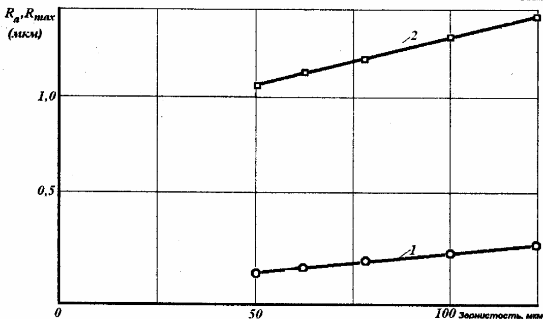
Рис. 3. Влияние зернистости абразива на интенсивность изменения значений высотных параметров шероховатости поверхности (режим обработки: давление 40 МПа; скорость резания 35 м/мин; продолжительность обработки 20 с): 1 – R_a ; 2 – R_{max} (до обработки R_a=0,68 мкм; R_{max}=3,64 мкм)
