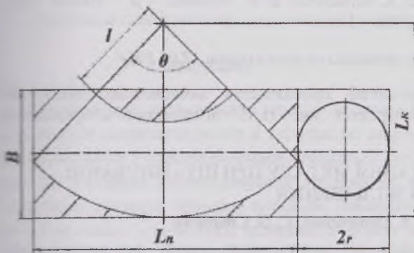
Рис. 3. Форма заготовки для изготовления конического полуфабриката
