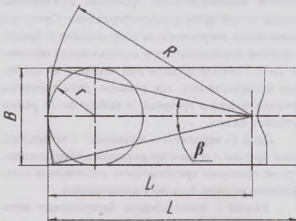
Рис. 1. Форма сектора заготовки
