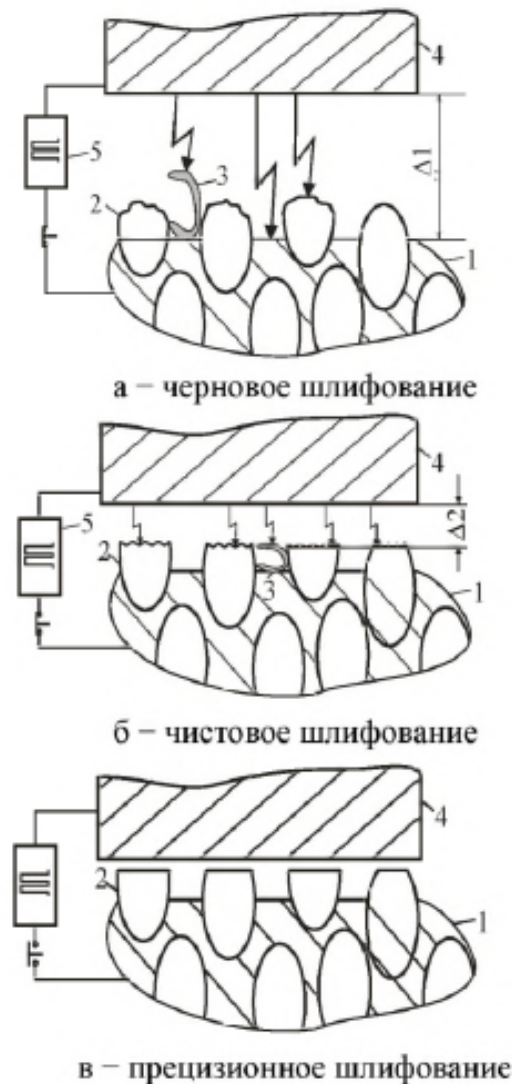
Рисунок – Способ комбинированной обработки материалов 1 – связка круга; 2 – алмазное зерно; 3 – стружка; 4 – электрод - инструмент; 5 – генератор импульсов
