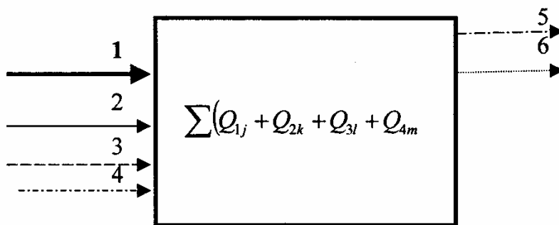
Рис. 1. Принципиальная схема энергопотоков в цехе (на предприятии): 1 – электроэнергия; 2 – сжатый воздух; 3 – гидропоток; 4 – топливо (горючий газ, жидкое топливо); 5 – вторично используемая энергия; 6 – безвозвратно потерянная часть энергии (из-за конвекции, излучения и др.); j, k, l, m – соответственно количество единиц оборудования в зависимости от вида подводимой энергии.
