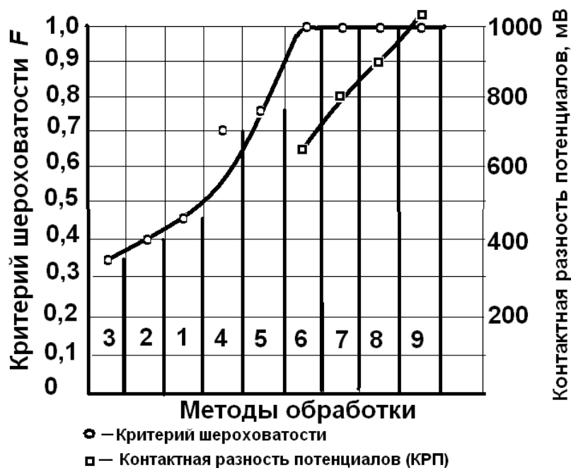
Рисунок 1 – Зависимость критерия шероховатости поверхности и КРП от методов обработки деталей из сплава АМгб: 1 – прокат; 2 – обработка металлической дробью; 3 – гидроабразивная обработка; 4 – фрезерование твердосплавной фрезой; 5 – фрезерование фрезой из эльбора; 6 – точение твердосплавным резцом; 7 – полирование алмазное; 8 – выглаживание; 9 – микроточение алмазным резцом
