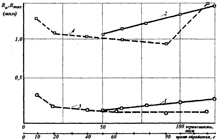
Рис. 1. Вплив зернистості абразивної стрічки 1, 2 і тривалості обробки 3 й 4 на інтенсивність зміни значень висотних параметрів шершкості поверхні (режим обробки: тиск 40 МПа; швидкість 35 м/хв; тривалість обробки 20 с. для 1 й 2; зернистість абразиву для 3 й 4 – АСО 50/40); 1, 3 – R_a ; 2 й 4 – R_{max}
