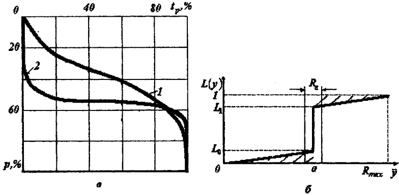
Рис. 2 – Відносні опорні криві поверхонь зразків з алюмінієвого сплаву марки АМг4 після обробки (а): 1- прокат (вихідна поверхня); 2 - абразивне полірування (б) - вид спрощеної функції L(\bar{y})
