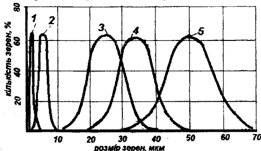
Рис.3. — Розподіл розмірів зерен алмазних мікро порошоків: 1 – АСМ 2/1; 2 – АСМ 7/5; 3 – АСМ 28/20; 4 – АСМ 40/28; 5 – АСМ 60/40
