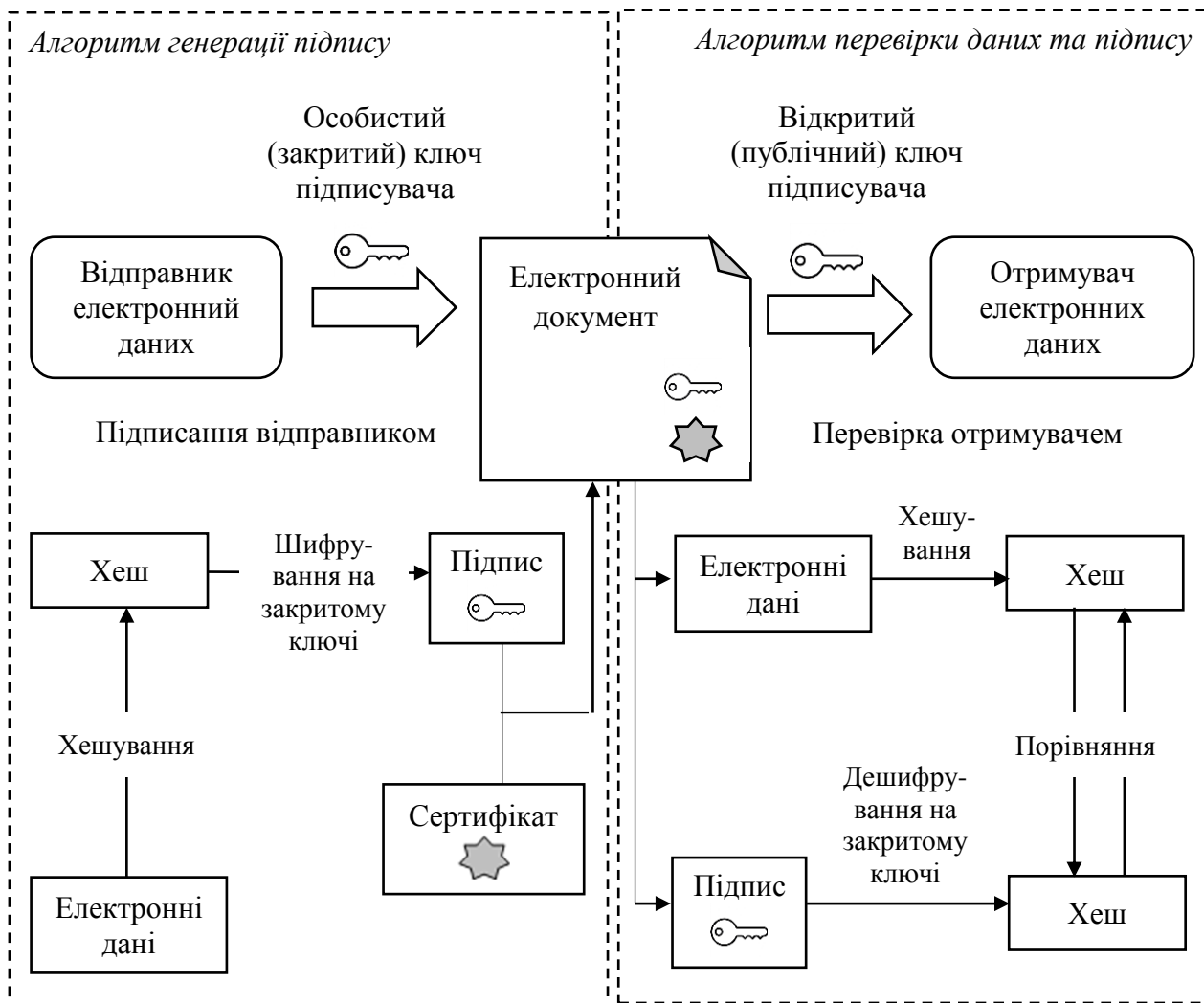
Рис. 1. Схема використання електронного цифрового підпису
