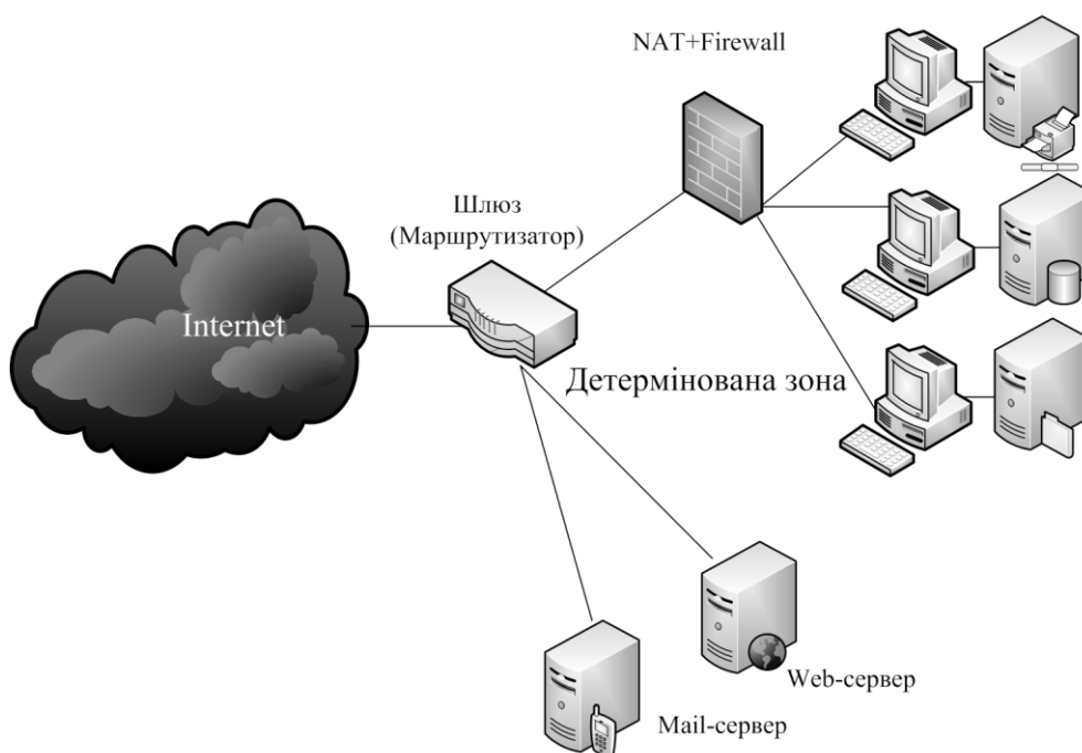
Рис. 23. Демілітаризована зона
