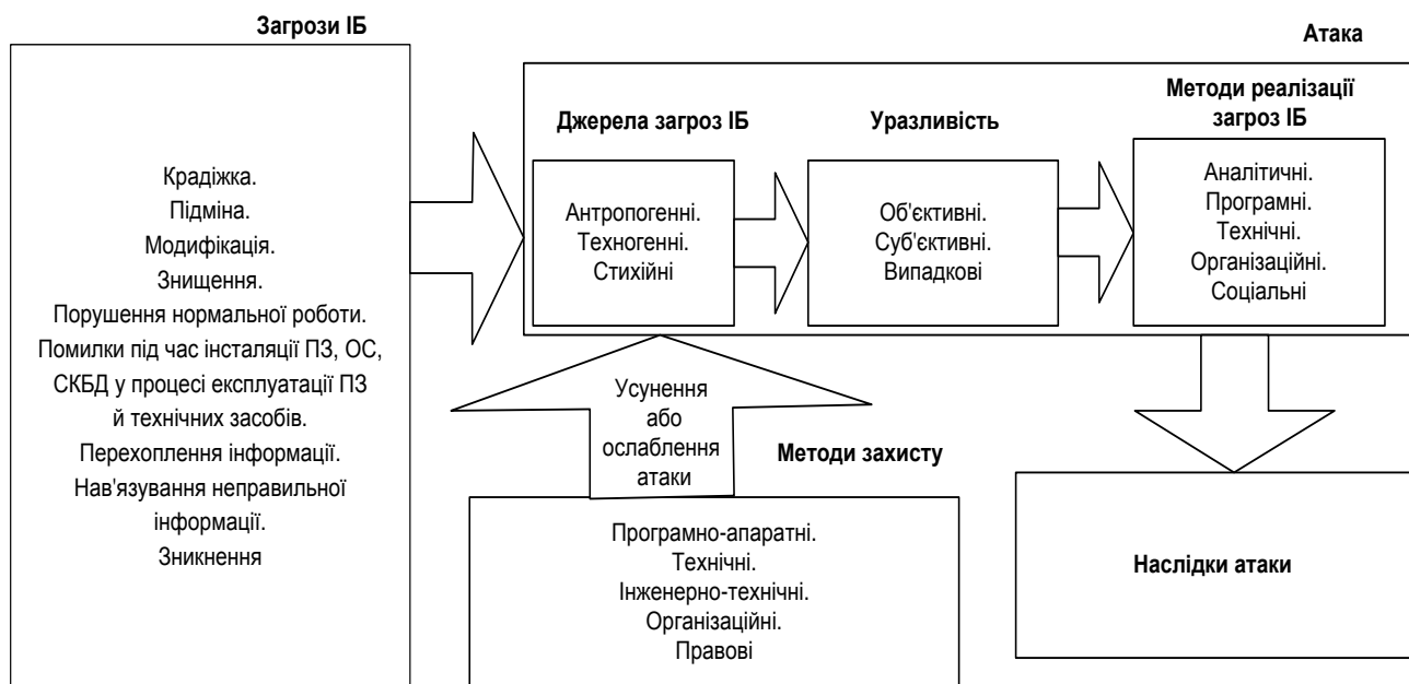
Рис. 7. Структурна схема моделі реалізації загроз інформаційних ресурсів у КміС
