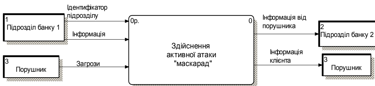
Рис. 15. Модель активних атак "маскарад"
