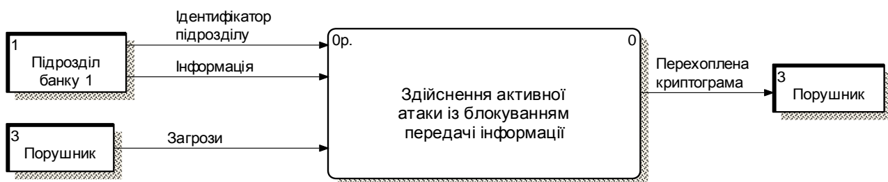
Рис. 11. Модель активних атак із блокуванням передавання інформації
