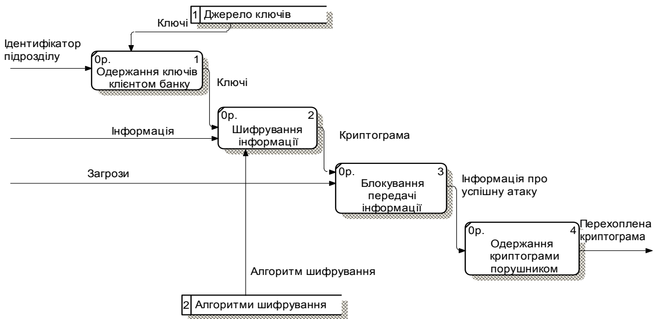
Рис. 12. Декомпозиція моделі активних атак із блокуванням передавання інформації
