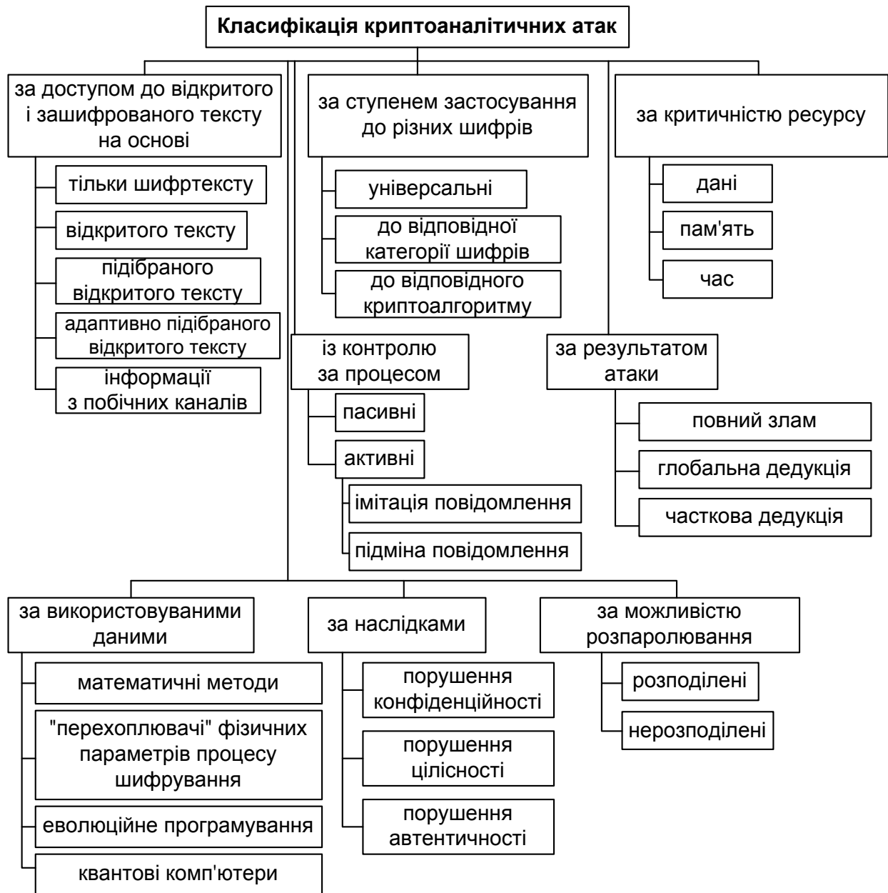
Рис. 3. Класифікація криптографічних атак
