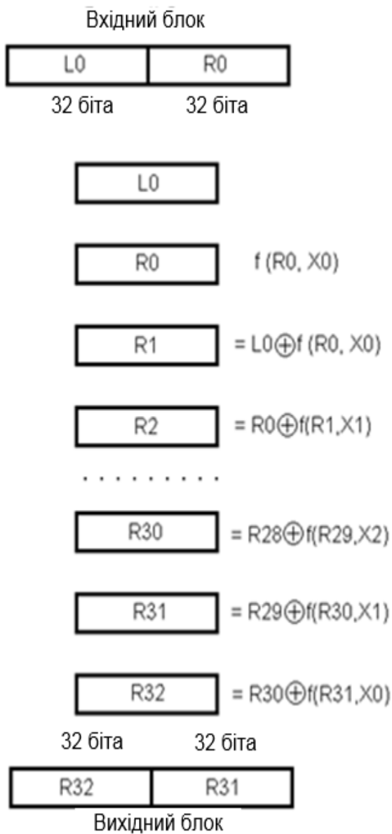
Рис. Б.1. Алгоритм шифрування ДСТУ 28147-89 (режим простої заміни)
