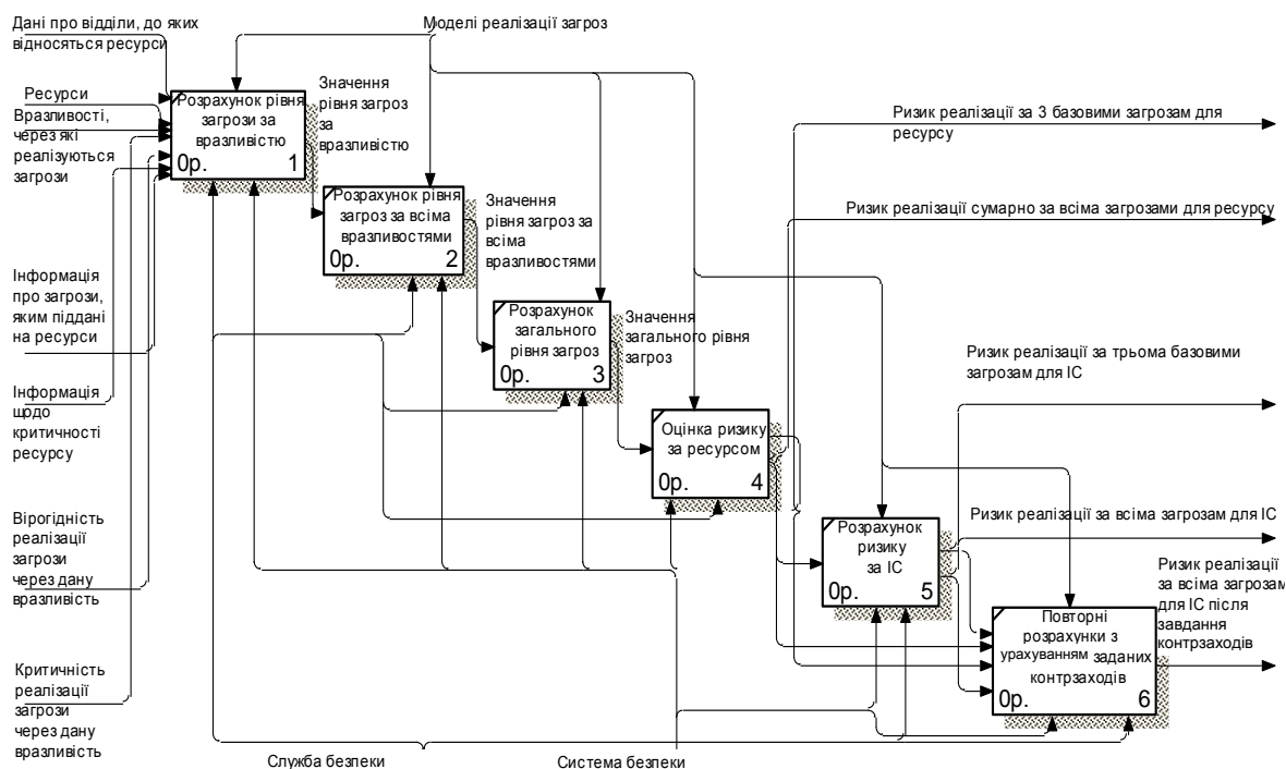
Рис. 18. Декомпозиція моделі оцінювання ризику реалізації загроз
