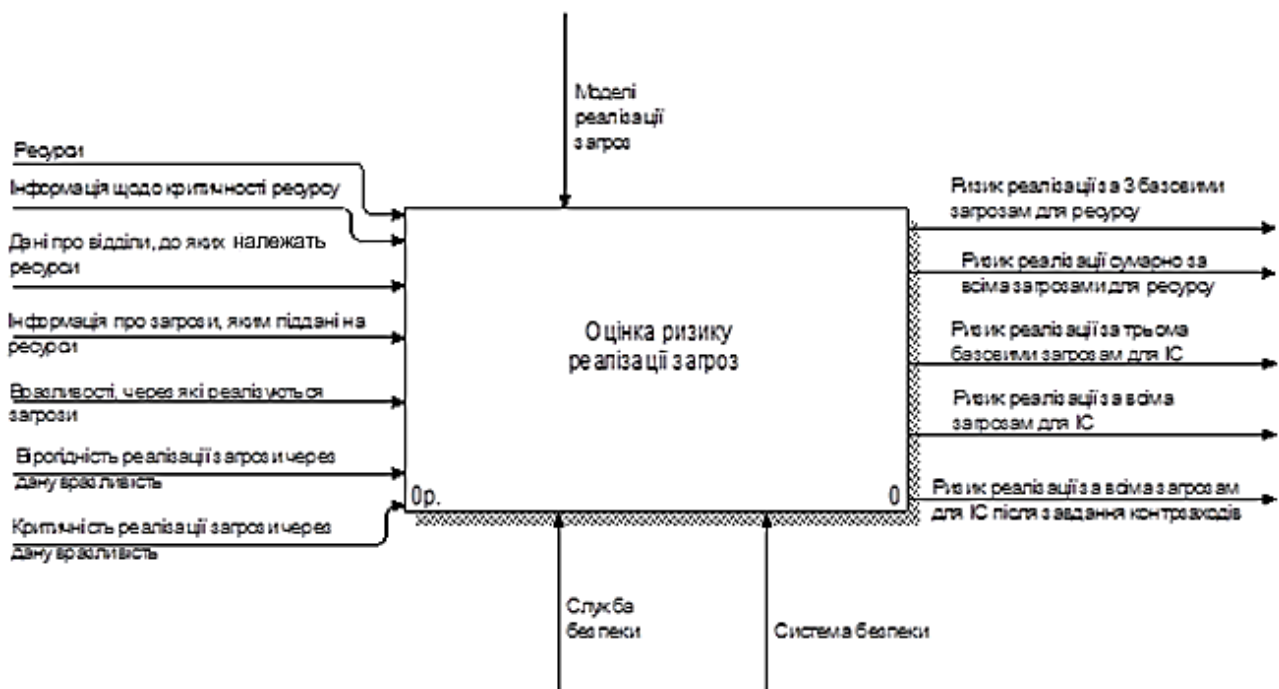
Рис. 17. Модель оцінювання ризику реалізації загроз (контекстна діаграма)
