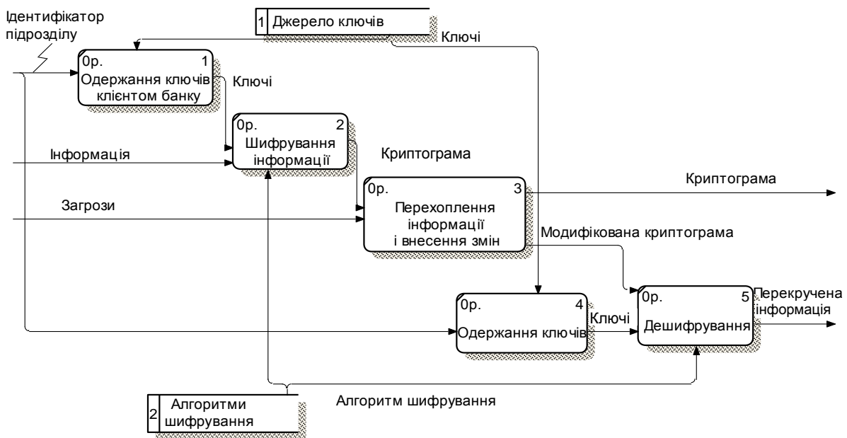
Рис. 14. Декомпозиція моделі активних атак із внесенням перешкод
