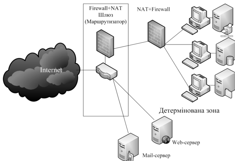
Рис. 21. Трансляція фіксованої внутрішньої адреси у фіксовану зовнішню
