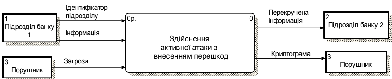
Рис. 13. Модель активних атак із внесенням перешкод
