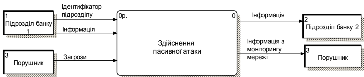
Рис. 9. Модель пасивних атак на інформаційні ресурси у КміС
