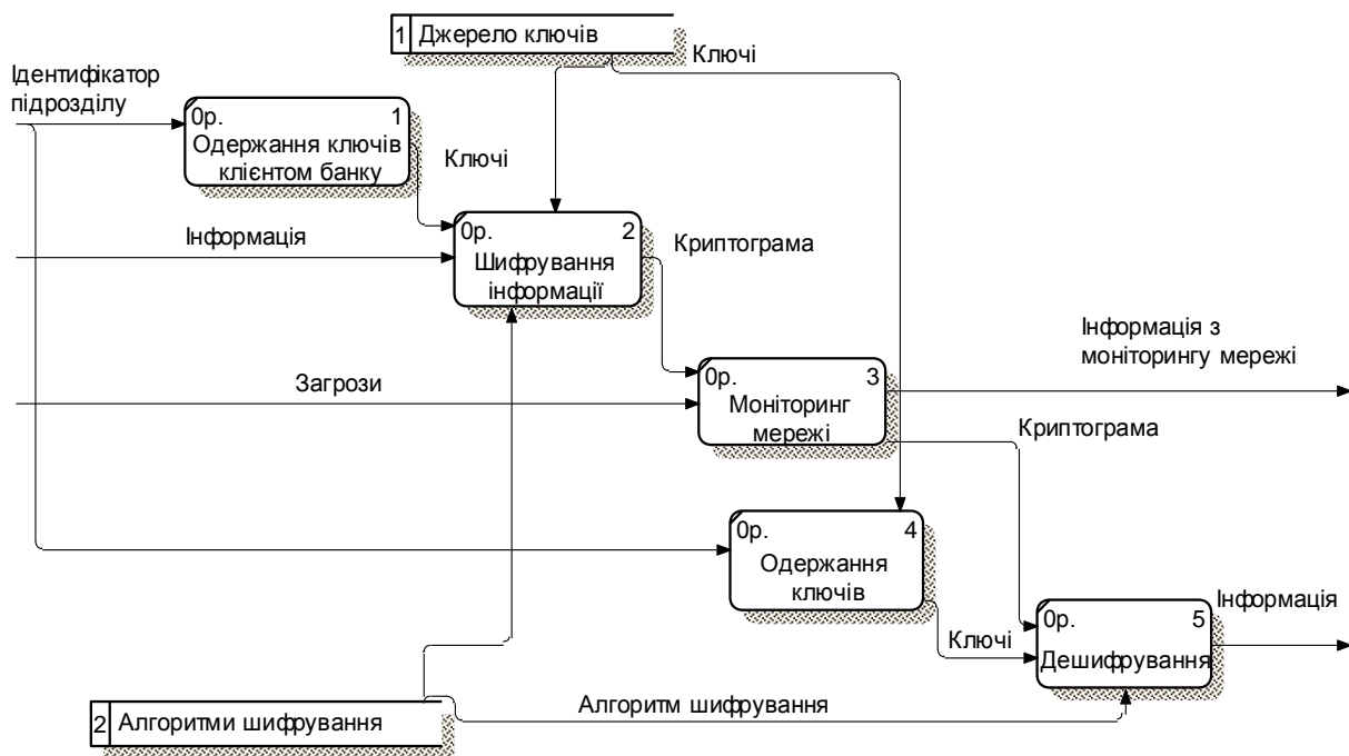
Рис. 10. Декомпозиція моделі пасивних атак
