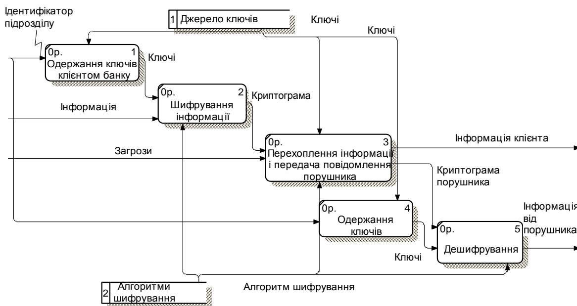
Рис. 16. Декомпозиція моделі активної атаки "маскарад"
