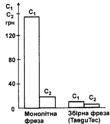
Рис. Діаграма розподілу витрат C_1, C_2 (на одну деталь) при фрезеруванні монолітною й збіркою фрезами
