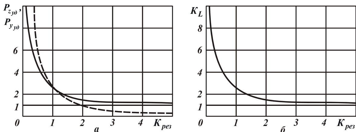
Рис. 1. Зависимости P_{z_{y\delta}} (сплошная линия) и P_{y_{y\delta}} (пунктирная линия)
