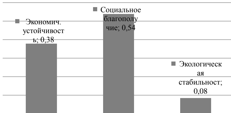
Рис. 2. Вектор приоритетов
