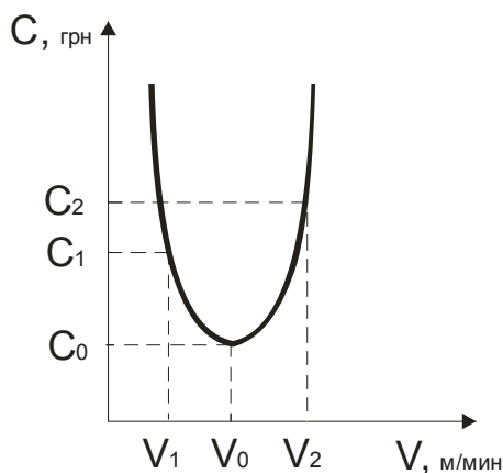
Рис. 2. Зависимость себестоимости обработки детали от скорости резания
