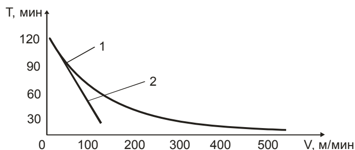
Рис. 1. Зависимость стойкости инструмента от скорости резания:
