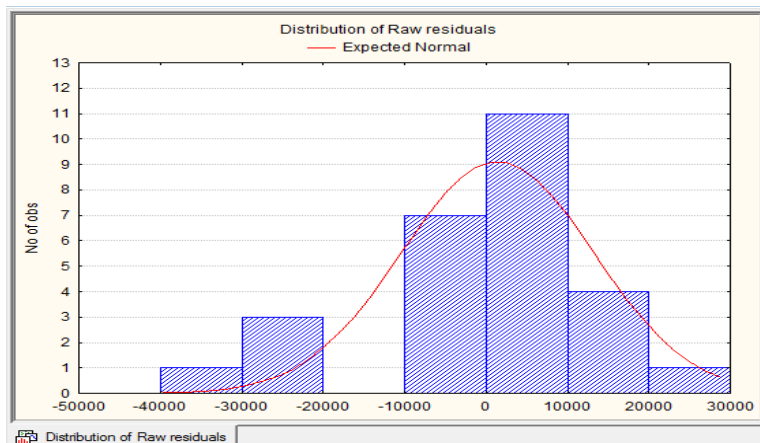
Рис. 16. Гістограма розподілу залишків
