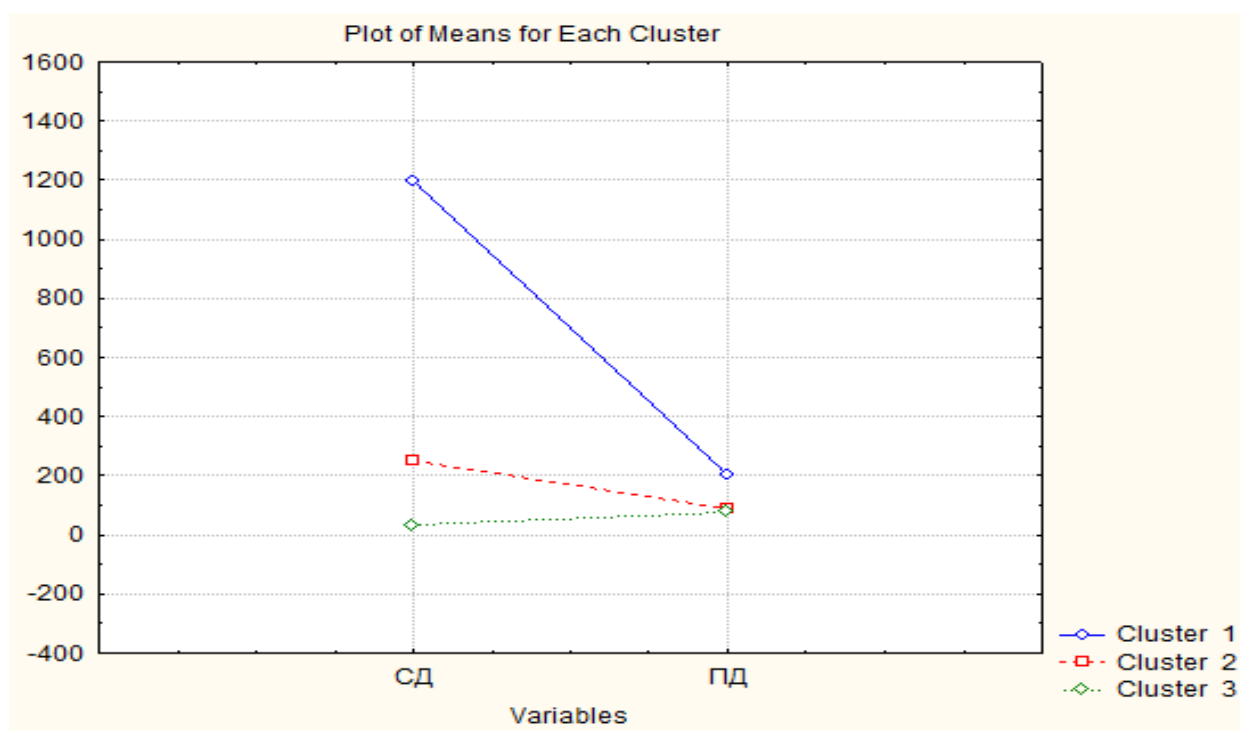
Рис. 25. Графік середніх значень показників для кластерів
