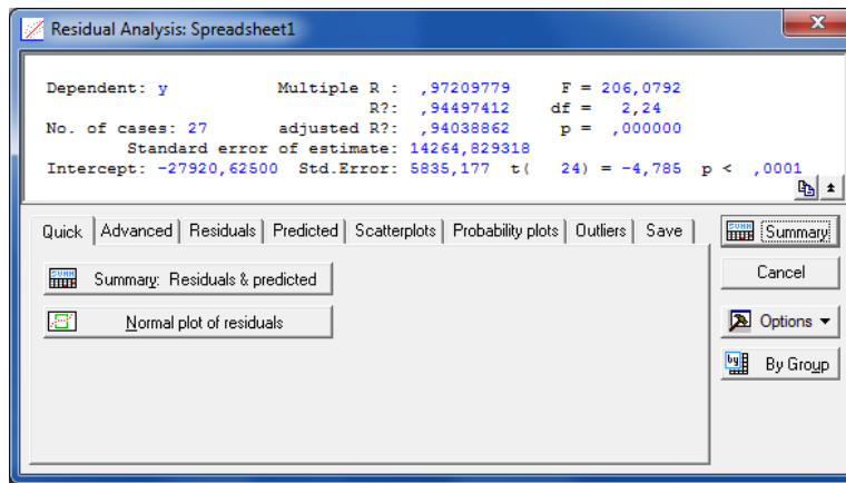
Рис.15. Вікно аналізу залишків
