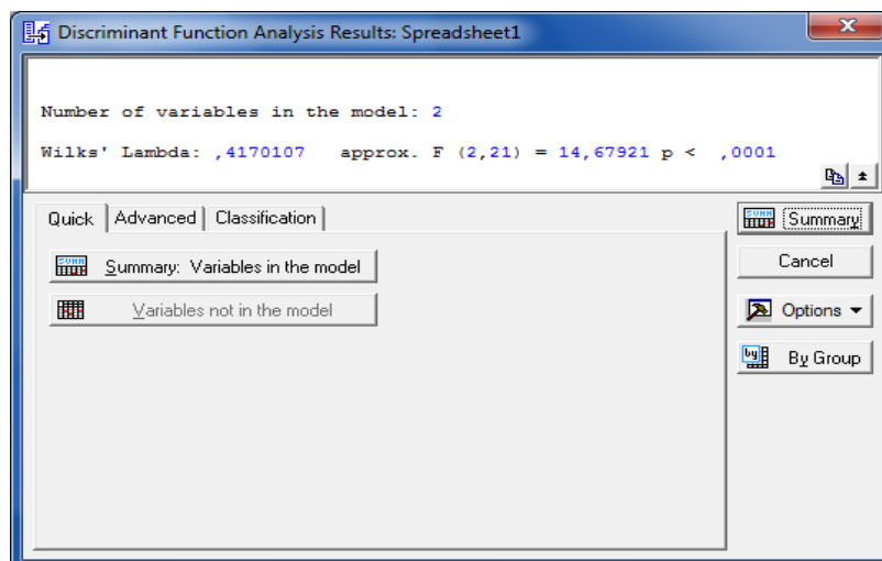
Рис. 28. Вікно "Результатів дискримінантного аналізу"
