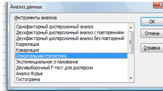
Рис. 3. Обрання режиму "Описова статистика"
