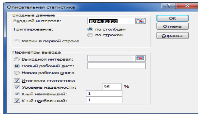
Рис. 4. Значення параметрів режиму "Описова статистика"
