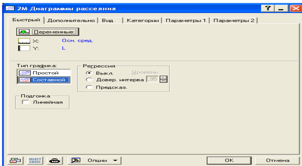
Рис. 40. Побудова ізокванти
