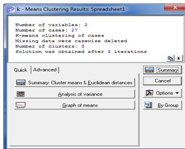
Рис. 24. Вікно результатів кластеризації методом k -середніх
