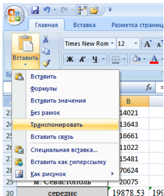
Рис. 50. Спеціальна вставка
