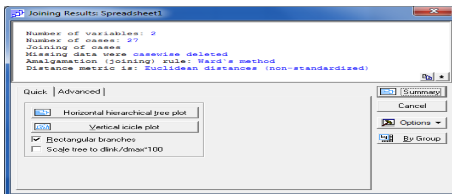
Рис. 21. Вікно результатів кластеризації ієрархічним методом
