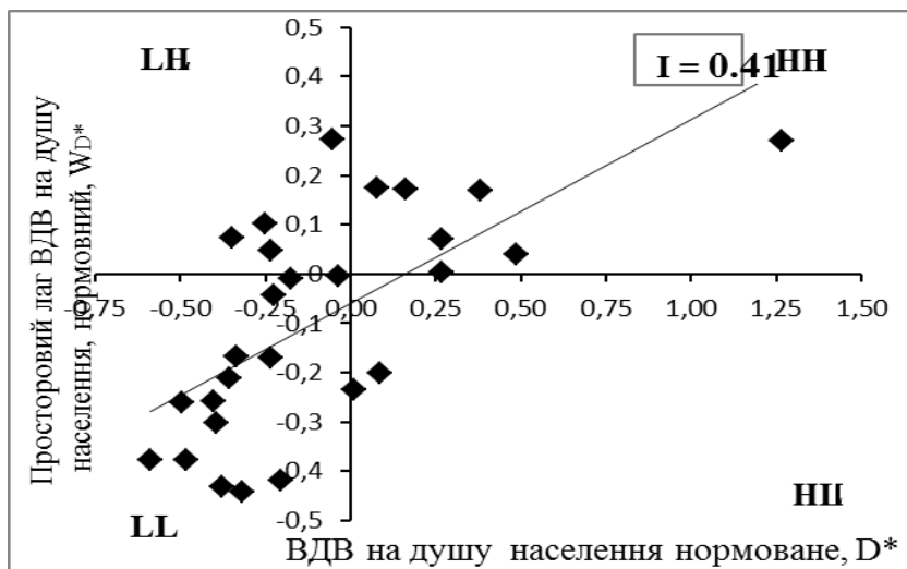
Рис. 53. Діаграма Морана
