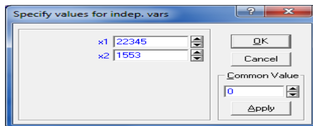
Рис. 18. Значення незалежних змінних для обчислення прогнозного значення залежної змінної
