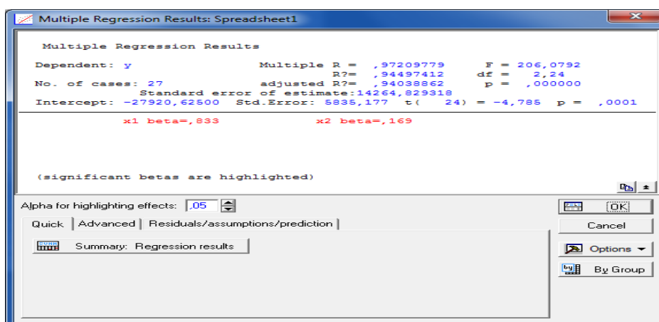
Рис. 13. Вікно результатів можинної регресії
