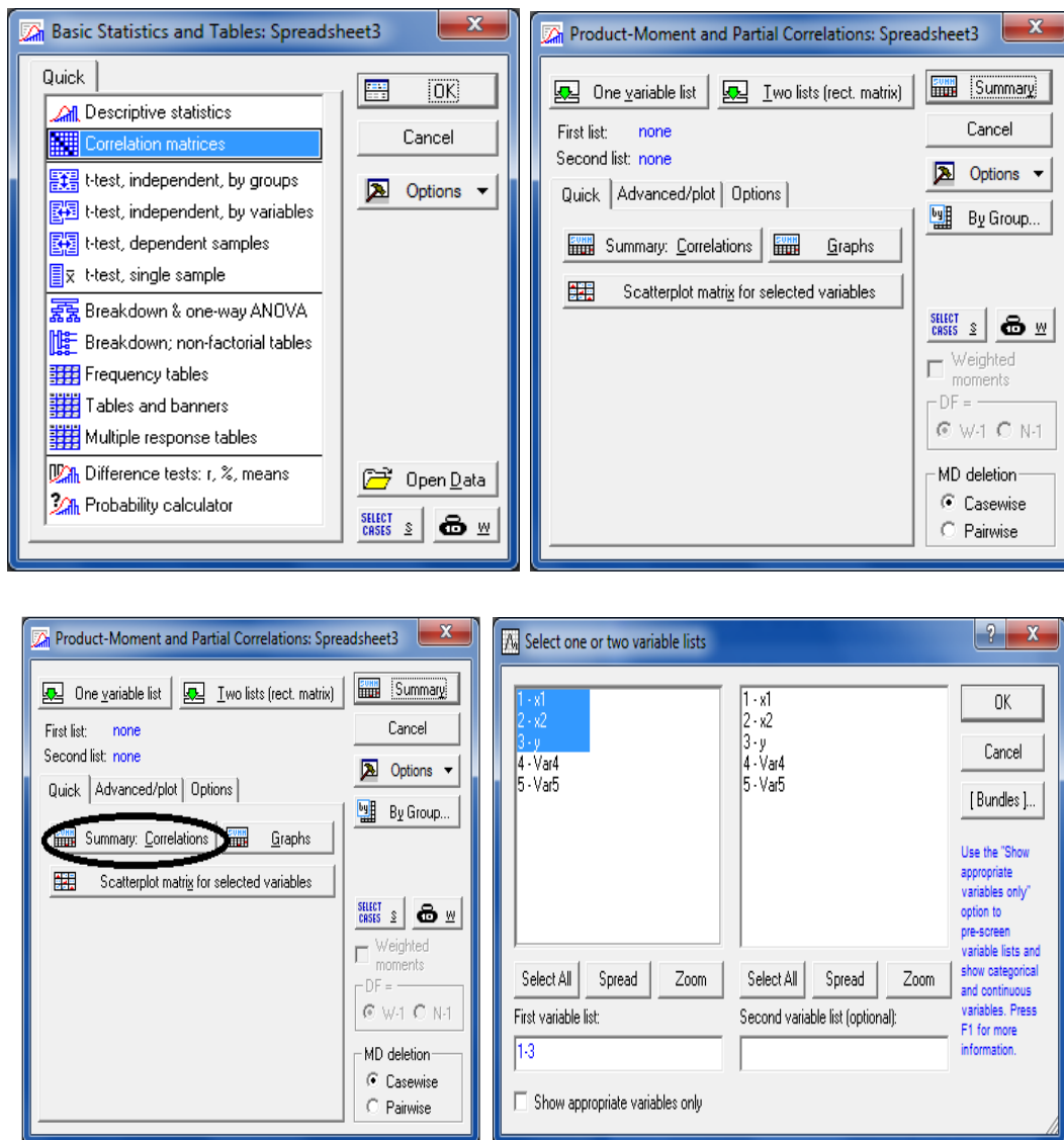
Рис. 11. Побудова кореляційної матриці
