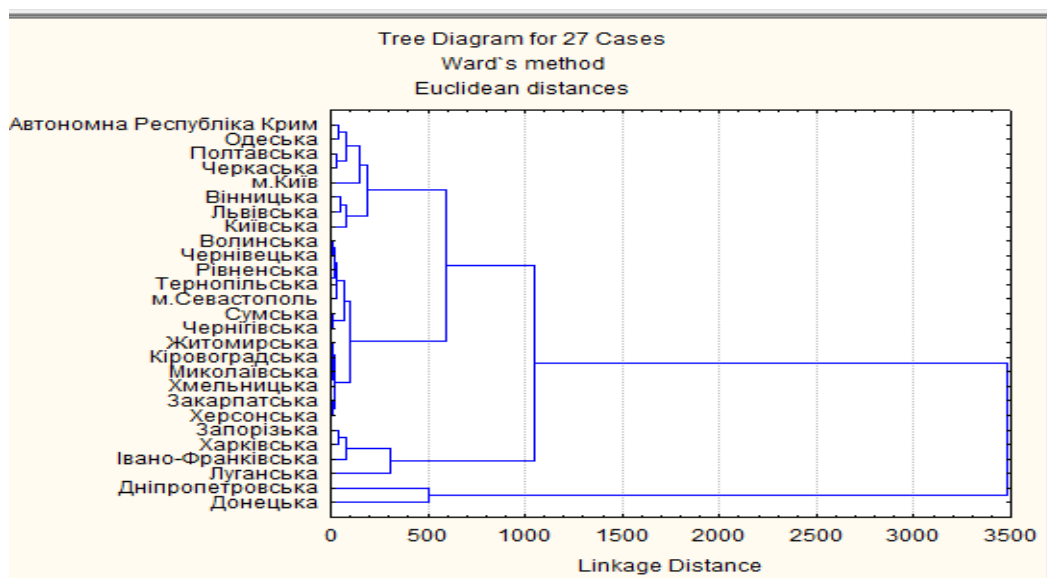
Рис. 22. Горизонтальна дендрограма
