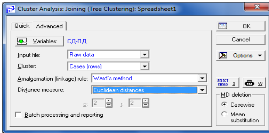
Рис. 20. Стартове вікно ієрархічного методу кластерного аналізу
