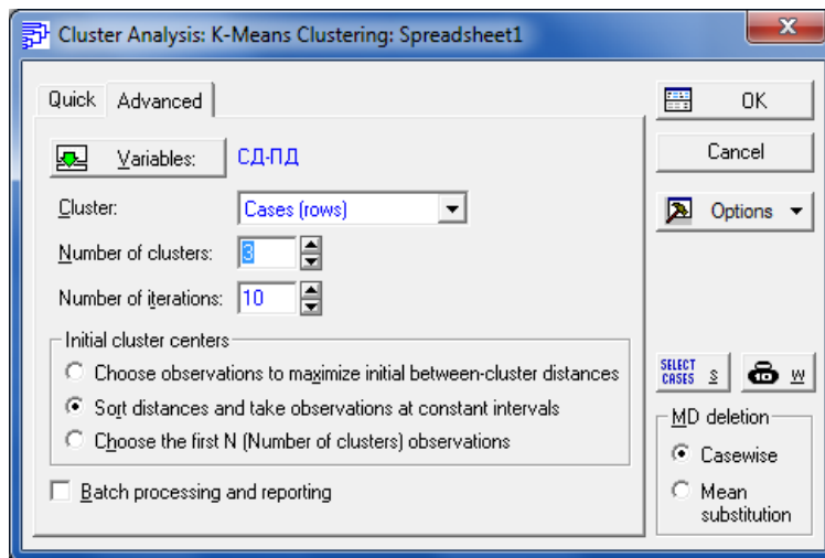
Рис. 23. Стартове вікно методу k -середніх
