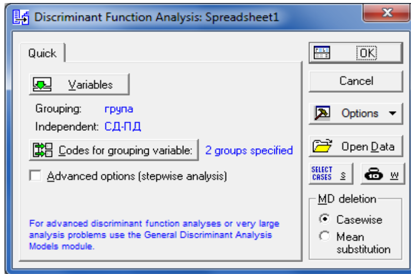
Рис. 27. Стартове вікно "Дискримінантного аналізу"
