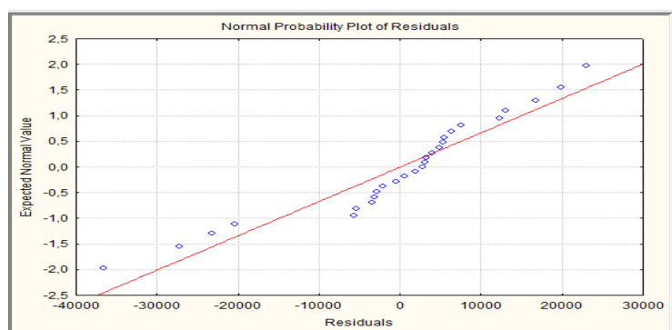
Рис. 17. Графік залишків на нормальному ймовірнісному папері
