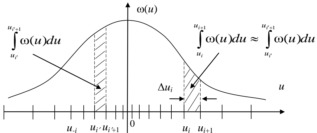
Рис. 4. Щільність розподілу ймовірностей випадкової неперервної величини u та зображення прикладу шкали, що забезпечує рівність ймовірностей при аналого-цифровому перетворенні – площ між поділками
