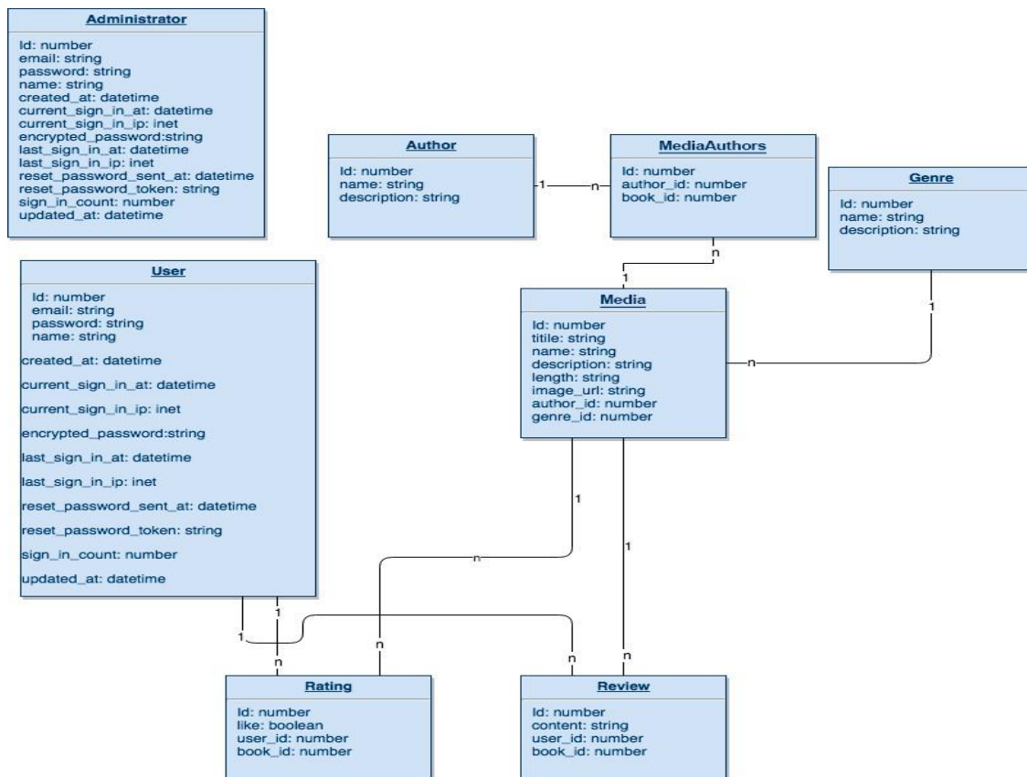
Рис. 4. Схема БД
