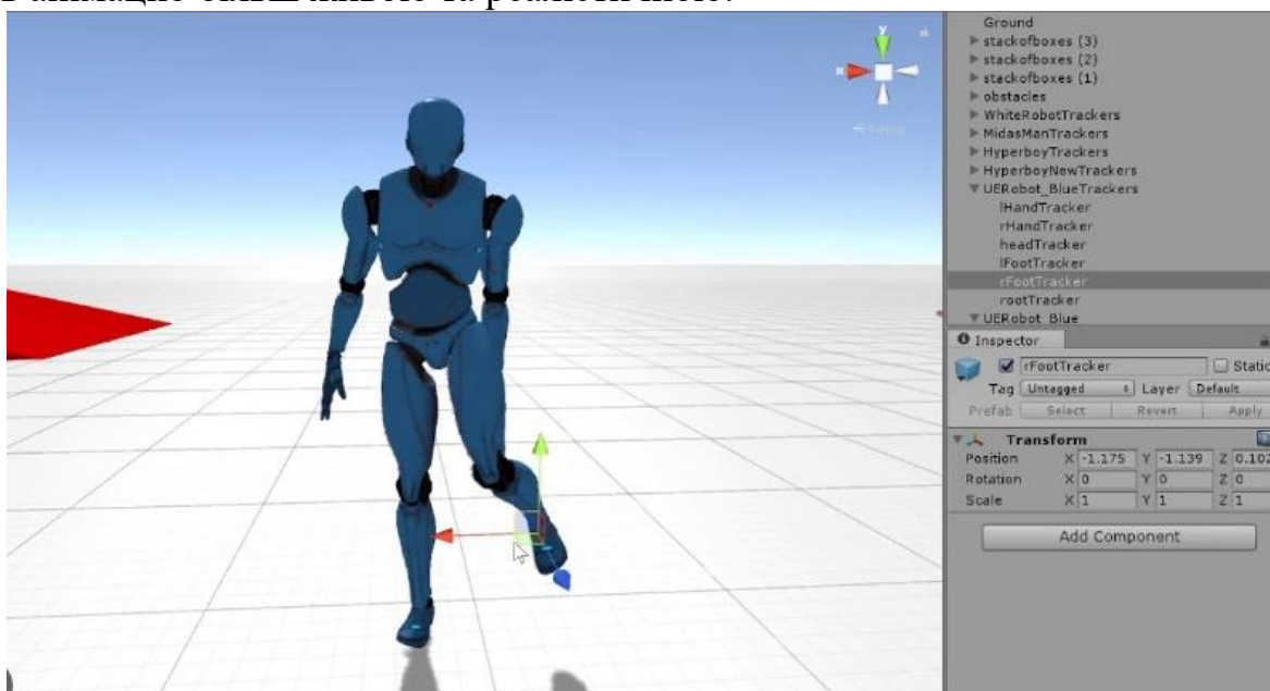
Рисунок 1 – DeepMotion Avatar
