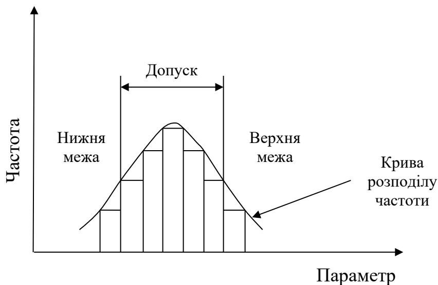
Рисунок 6.14 – Гістограма
