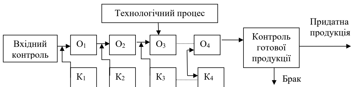
Рисунок 3.4 – Схема регулювання якості у процесі виробництва за допомогою статистичного контролю:
