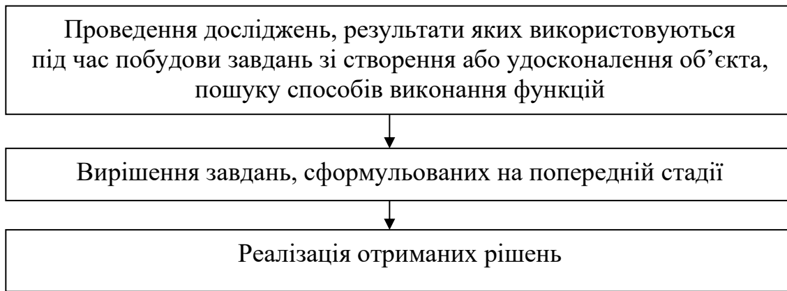
Рисунок 6.18 – Алгоритм ФВА
