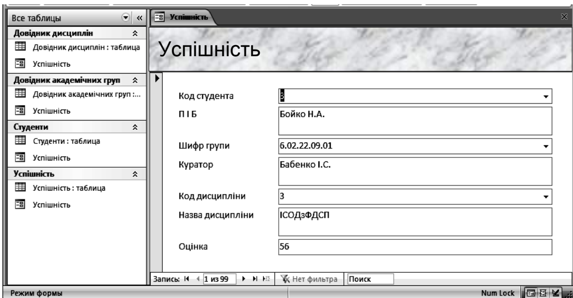
Рис. 5.21. Форма "Успішність"
