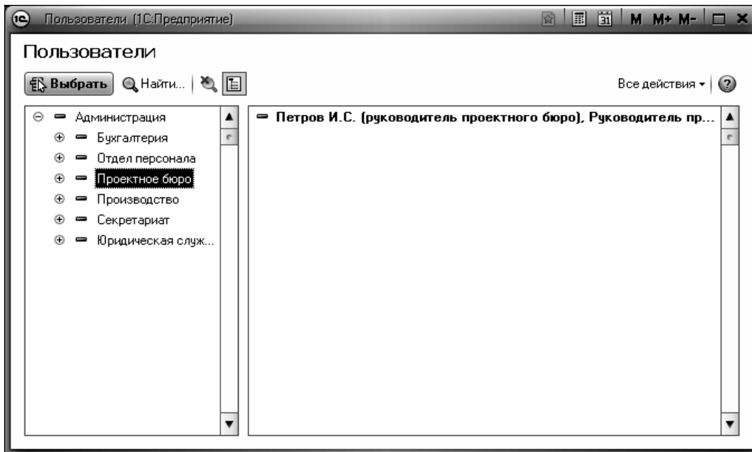
Рис. 9.9. Список користувачів
