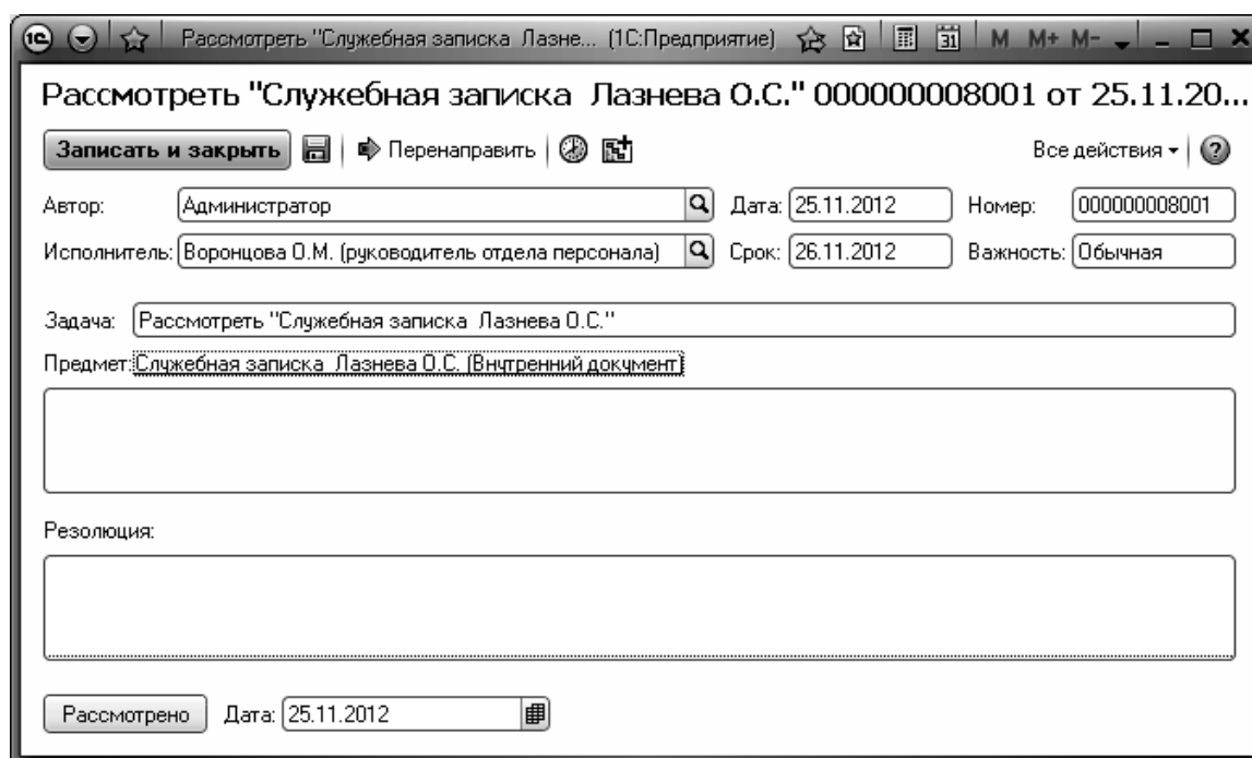
Рис. 9.6. Відкриття документа
