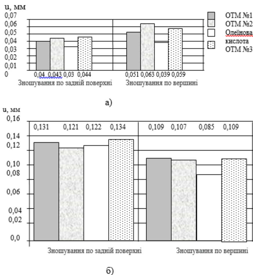
Рис. 1. Залежність зношування свердл від пройденого шляху: а) сталь марки ШХ15; б) сталь марки X18Н9Т
