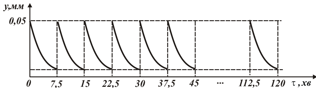
Рис. 10. Характер зміни величини пружного переміщення y в технологічній системі від часу обробки \tau
