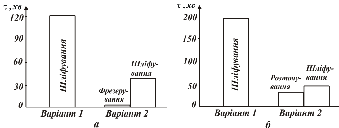
Рис. 9. Діаграма розподілу машинного часу обробки для двох варіантів технологічного процесу обробки отворів у кільцях з магнітного сплаву твердістю HRC 62 – 63 (а) і твердістю HRC 56 – 58 (б)
