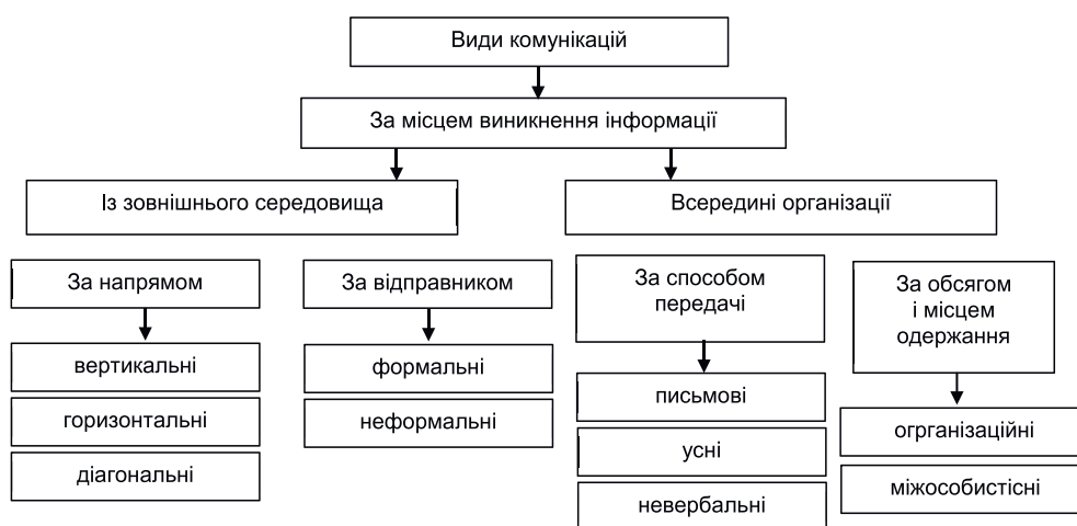
Рис. 1. Види комунікацій
