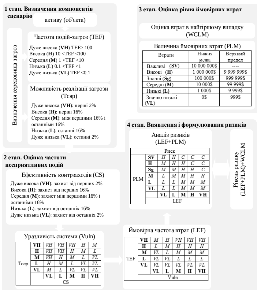
Рис. 3 Методика оцінки ризиків FAIR
