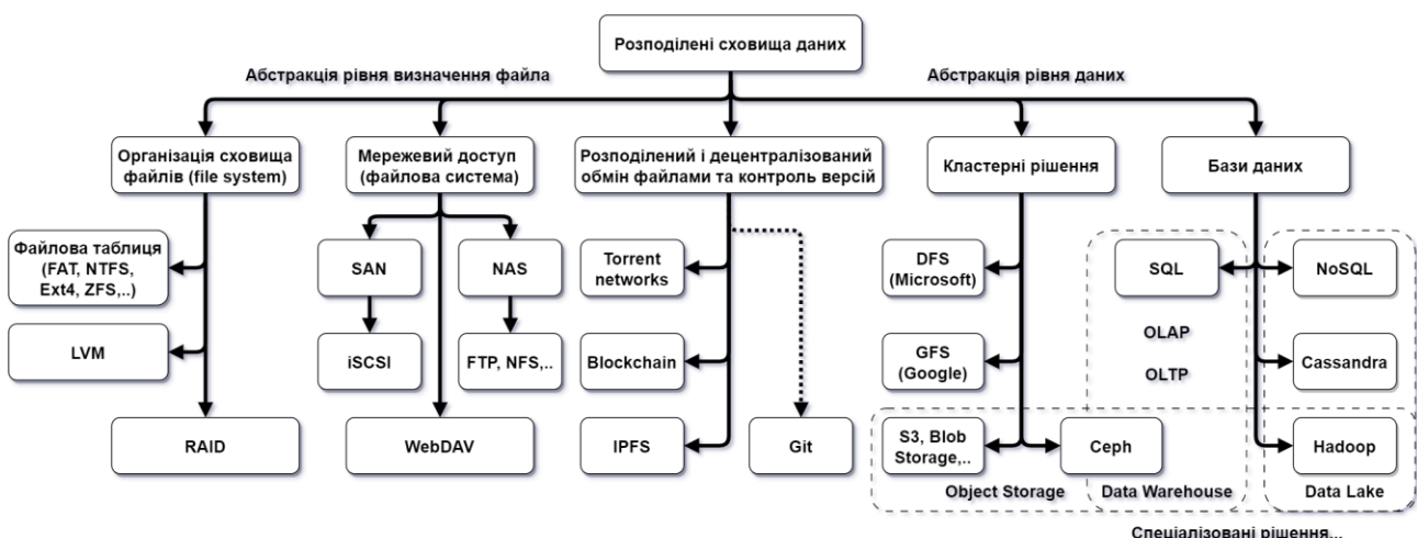
Рисунок 1 – Технології побудови сховищ даних
