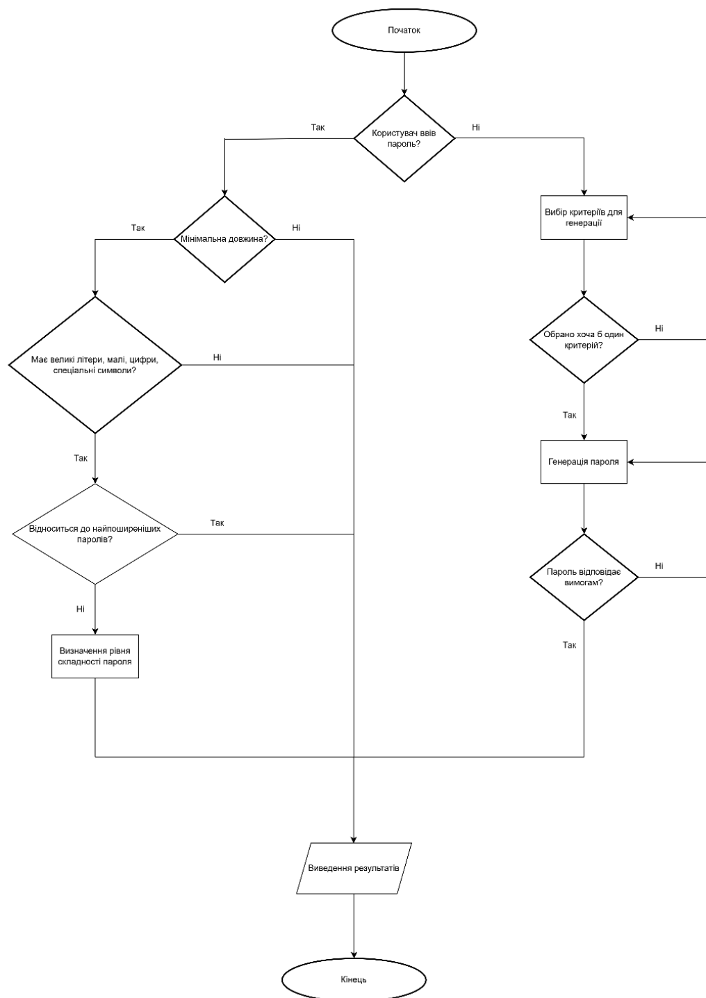
Рисунок 2. Алгоритм роботи вебсервісу
